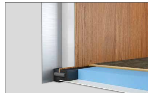
+ Kosteutta kestävä lattiarakenne on suojattu lasikuitulevyllä
