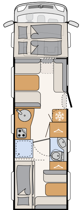
XXL A 9000-2 K
